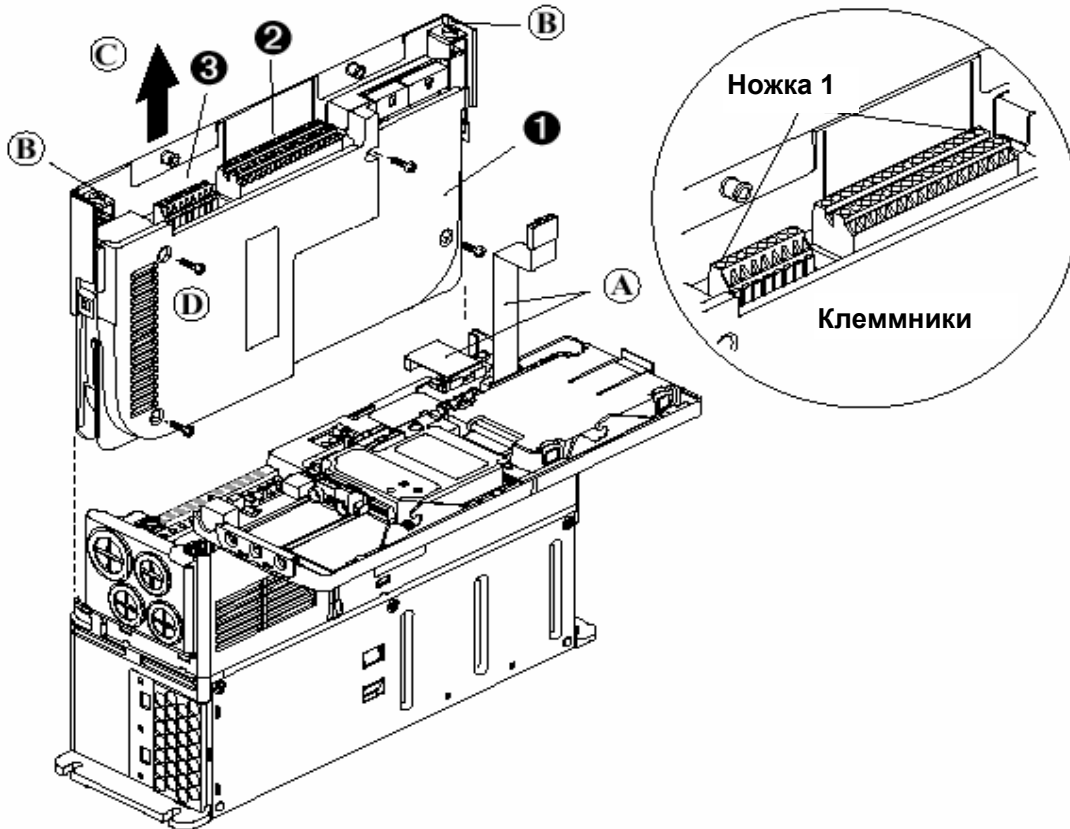
Рис. 1.6 Типичная кассета и клеммники ввода/ вывода PowerFlex 700
