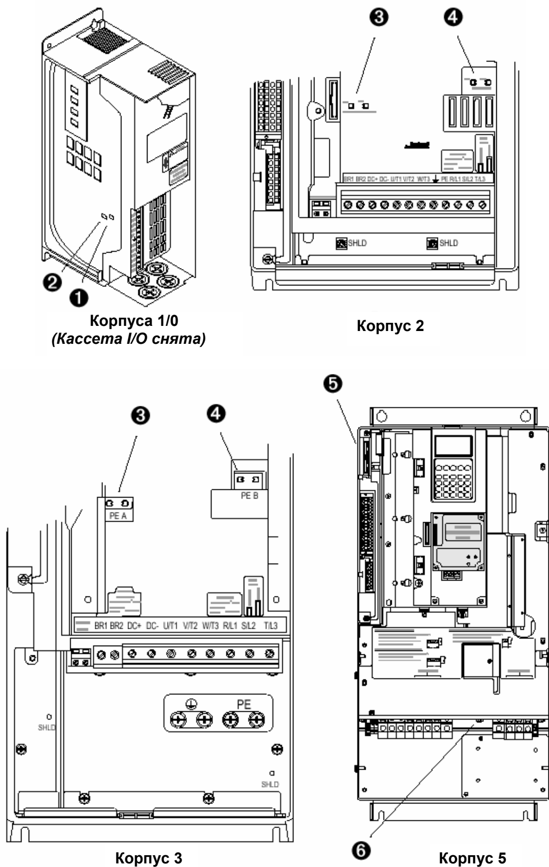
Рис. 1.5 Стандартное расположение перемычек (См. описание в таблице 1.D )
