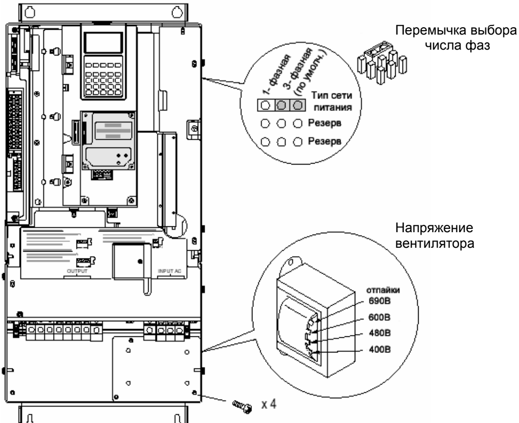
Рис. 1.2 Расположение переключки и трансформатора в приводах типа 5
