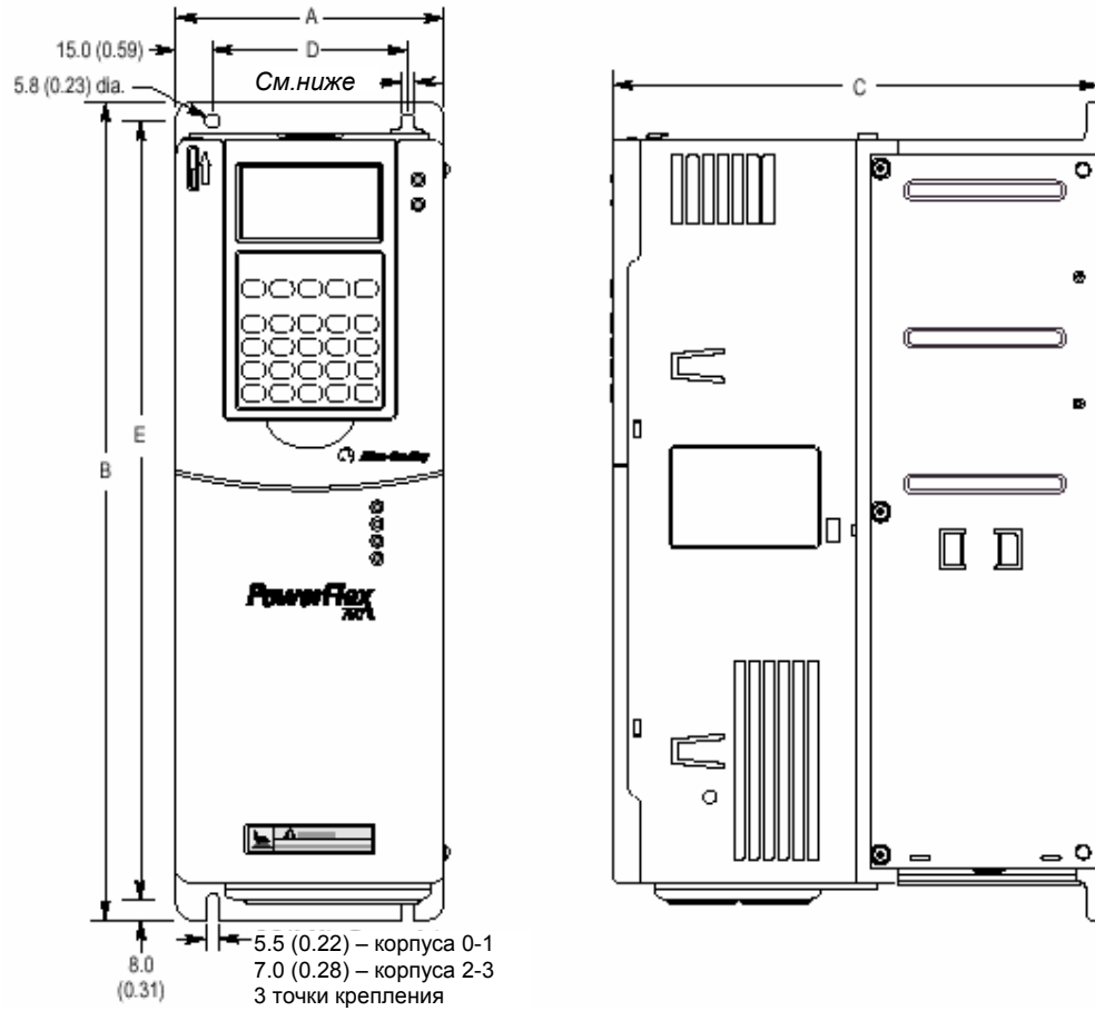
Рис. А.3 Корпуса типов 0-3 приводов PowerFlex 700 (Показан корпус 0)
