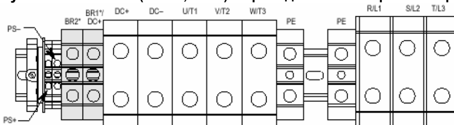
Корпус 5 – 100 л.с. 480В – привод с обычным режимом работы
