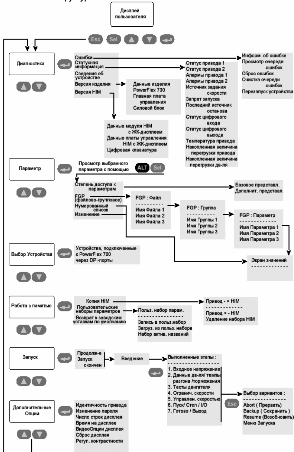
Рис. В.1 Структура меню HIM
