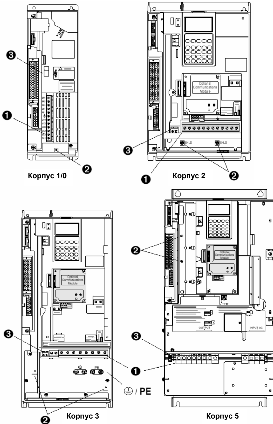
Рис. 1.3 Типичное расположение силового клеммного блока
