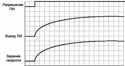
Преде.уставка ПИ = 0
