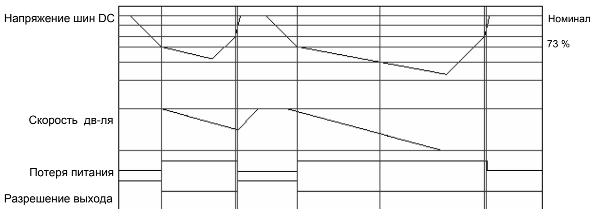
Рис. С.2 Режим Потери Питания = Самовыбег
