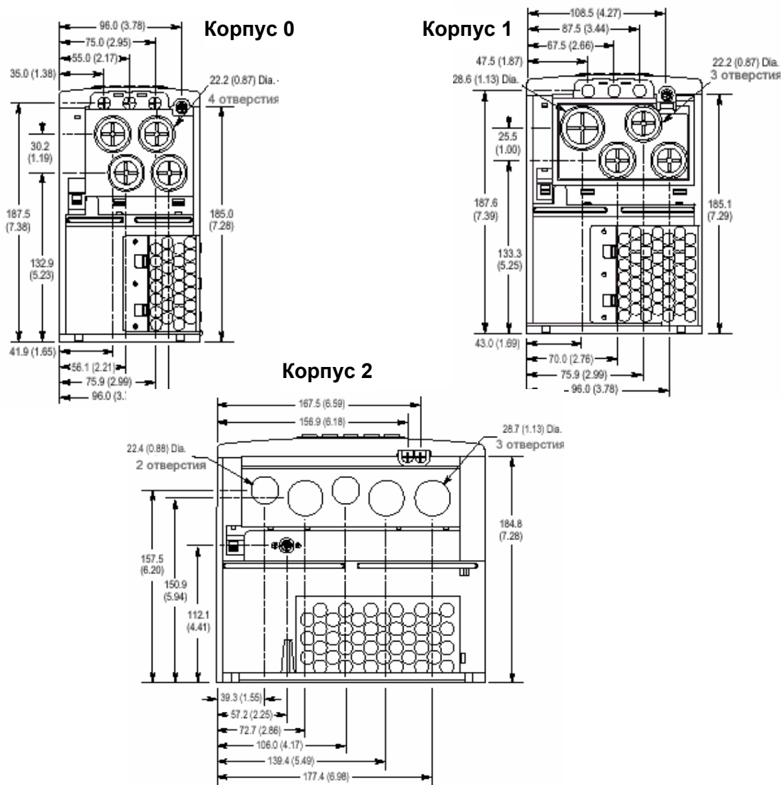
Рис. A.5 Размеры приводов PowerFlex 700 - Вид снизу
