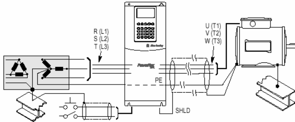
Рис. 1.1 Типичная схема заземления
