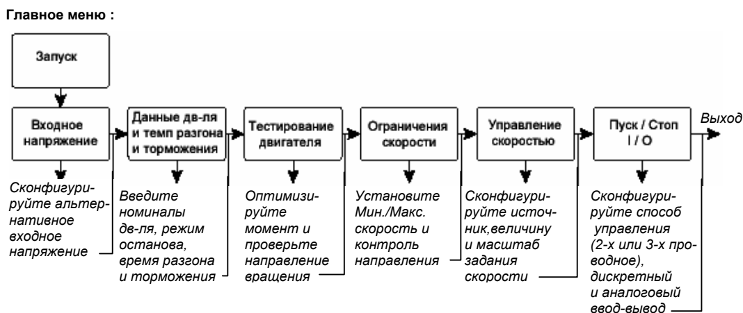
Рис. 2.2 Меню запуска при опции обычного управления
