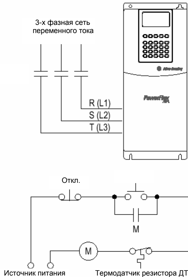
Рис. С.1 Цепь внешнего резистора торможения
