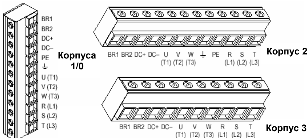
Рис. 1.4 Силовой клеммный блок
