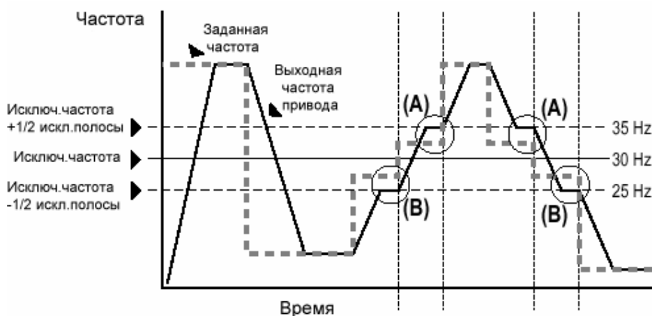
Рис. С.6 Исключаемая частота
