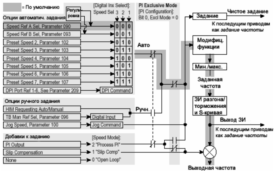
Рис. 1.10 Диаграмма выбора задания скорости (1)
