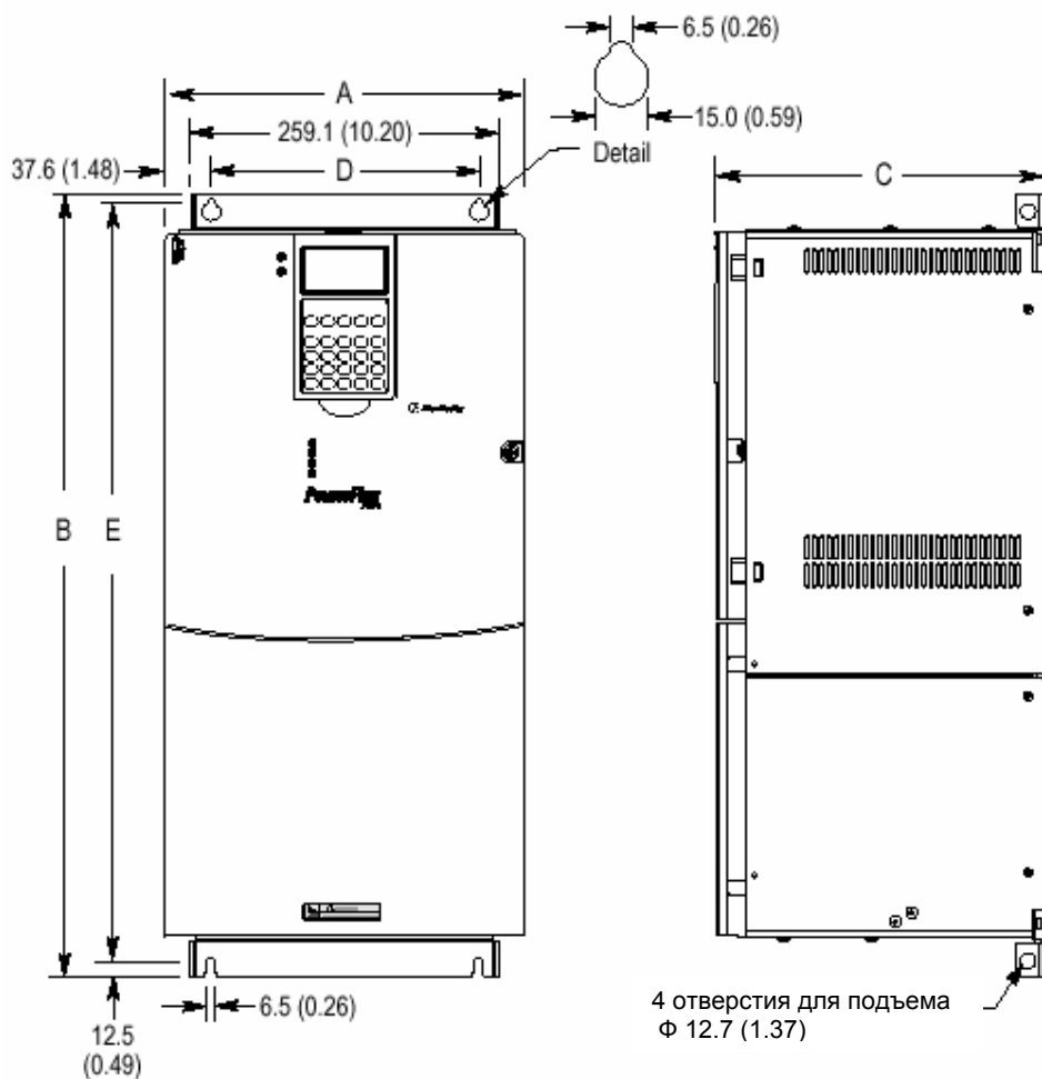
Рис. А.4 Корпус типа 5 приводов PowerFlex 700
