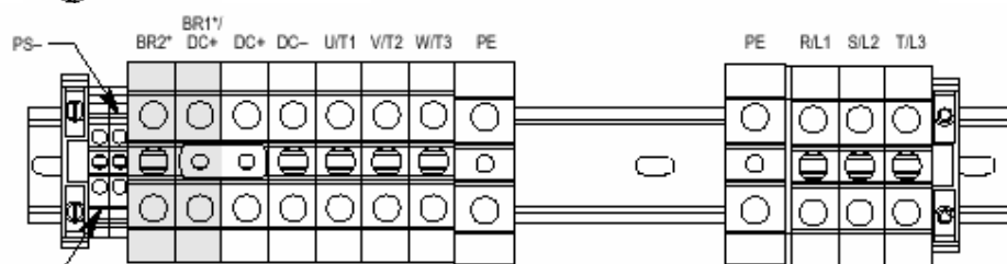
Корпус 5 – 75 л.с. 480В (55КВт, 400В) – привод с обычным режимом работы
