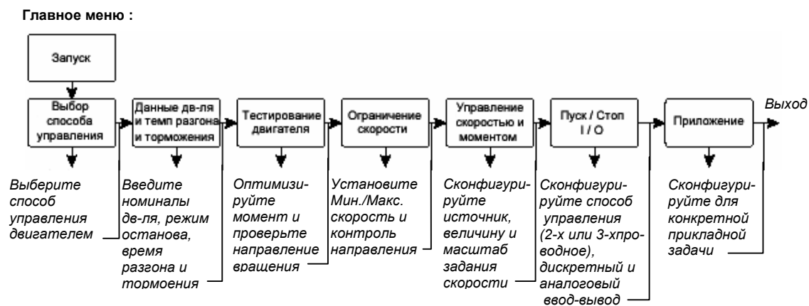
Рис. 2.3 Меню запуска при опции векторного управления
