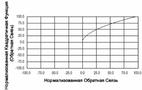
Преде.уставка ПИ > 0
