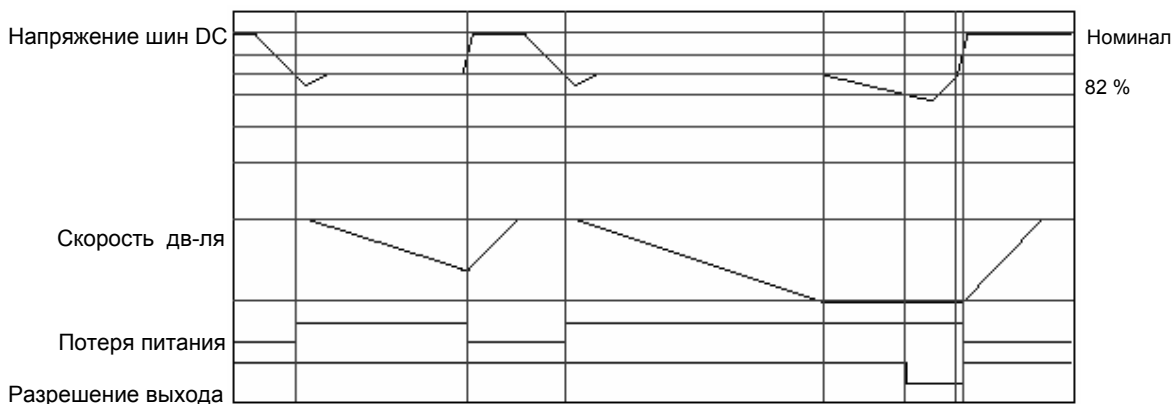
Рис. С.3 Режим Потери Питания = Торможение
