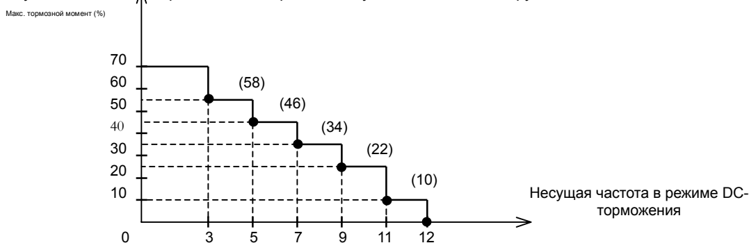
Ограничение тормозного момента в зависимости от значения несущей частоты
