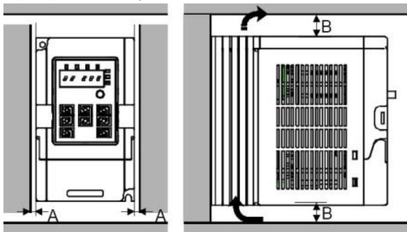
Рис. 3-2 Место установки
