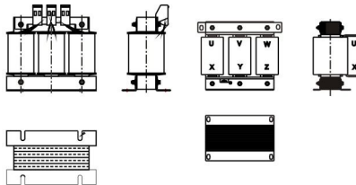
Входной реактор
