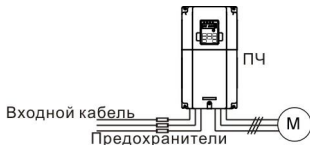
Рис.3-10 Подключение предохранителей
